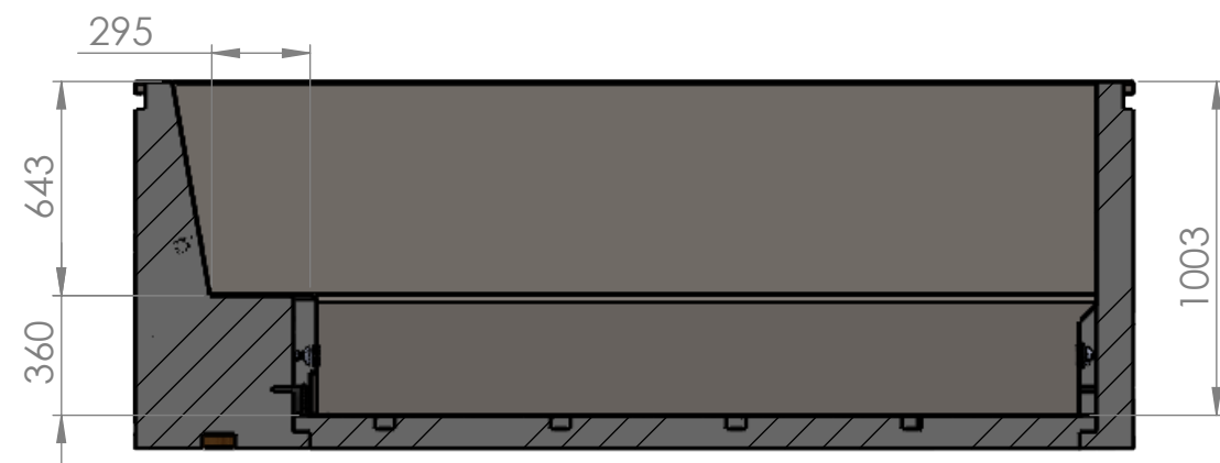
SECTION D-D SCALE 1 : 25
